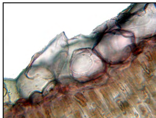
Figure 8. Micrograph of cross section through the lamina of Halimione verrucifera (X400). / Figura 8. Secțiune transversală prin limbul foliar de la Halimione verrucifera (X400) (original).
